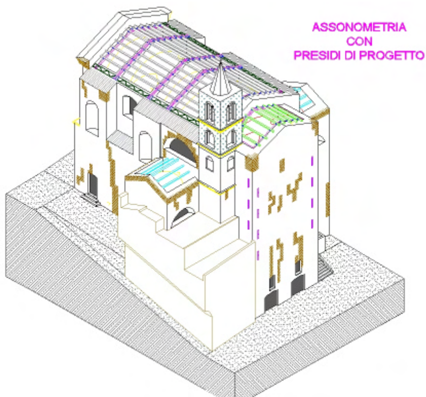
Figura 1. Ricostruzione tridimensionale dell'intervento
