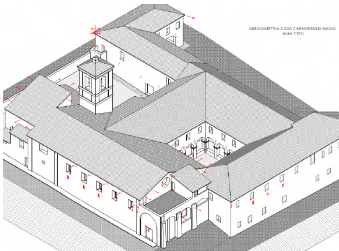
Figura 4. Assonometria con i cinematismi di danno
