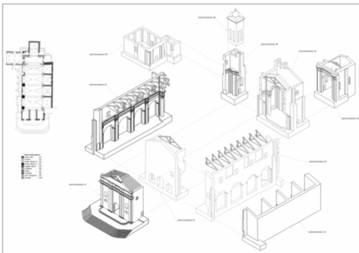
Figura 2. Suddivisione in macroelementi
