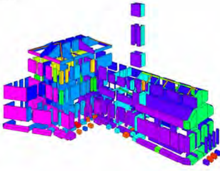
Figura 14. Verifiche strutturali dei setti murari
