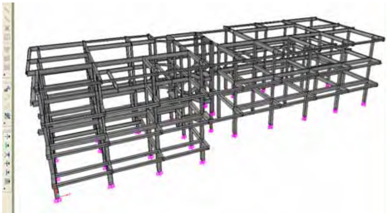
Figura 7. Verifiche strutturali di edifici esistenti in c.a.
